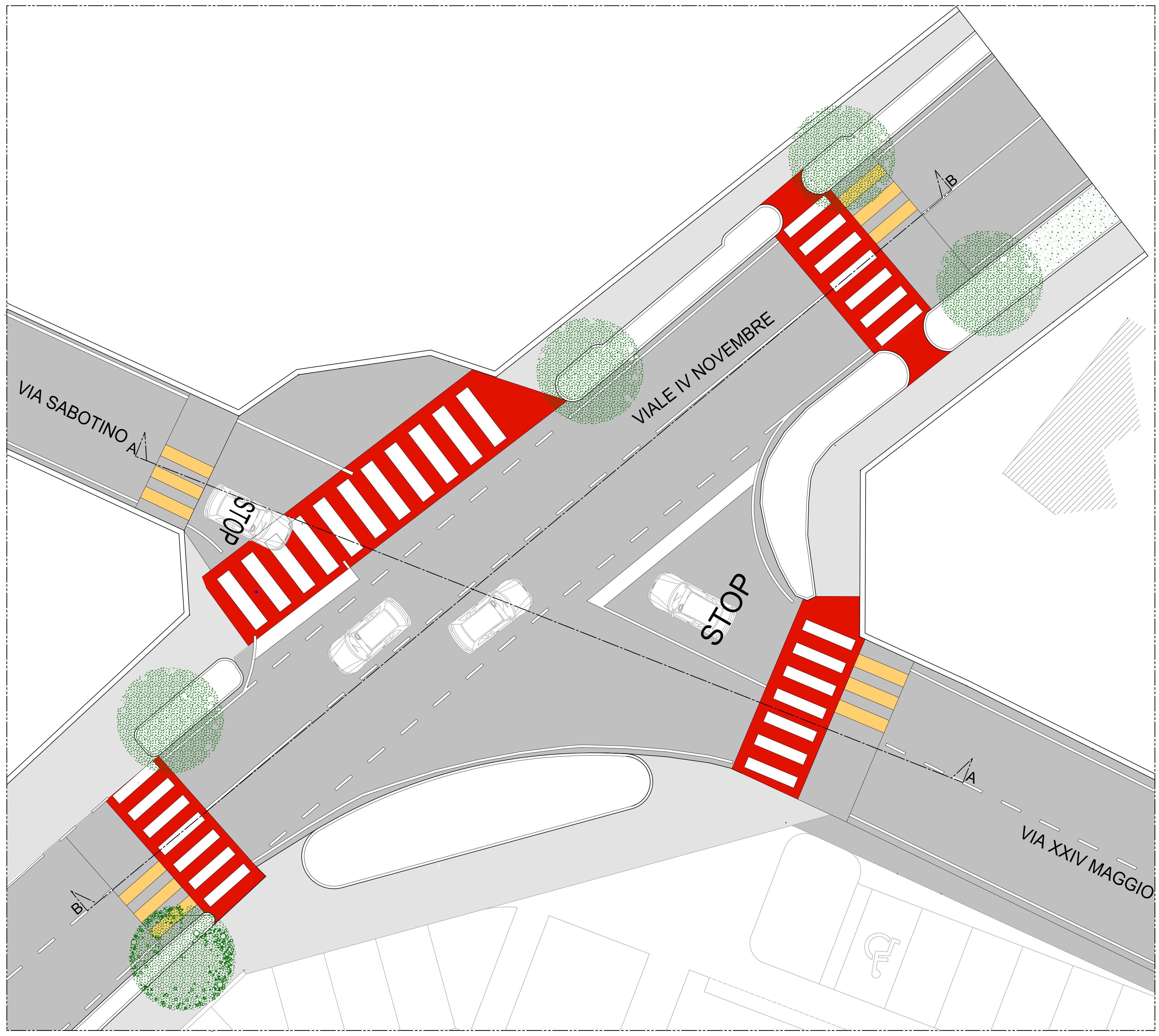
PIANTA DI PROGETTO INTERSEZIONE DA RIQUALIFICARE scala 1:200
