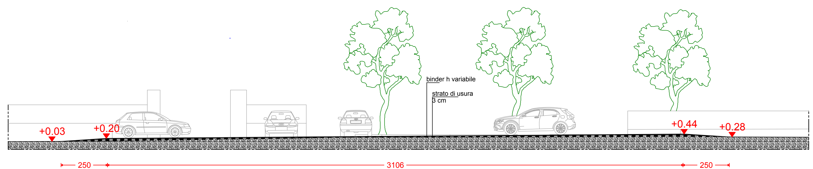
SEZIONE AA DI PROGETTO INTERSEZIONE DA RIQUALIFICARE scala 1:200
