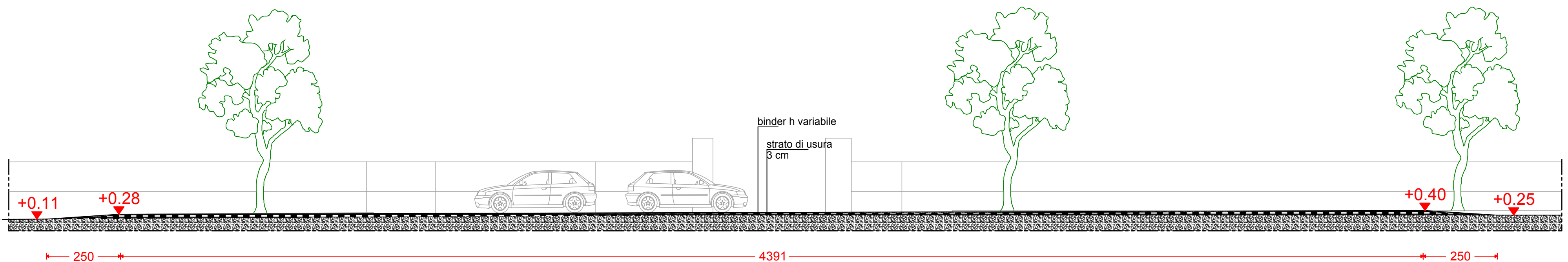
SEZIONE BB DI PROGETTO INTERSEZIONE DA RIQUALIFICARE scala 1:200
